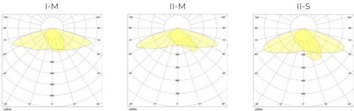
KRZYWE ROZSYŁU / LIGHT BEAM CURVES:
